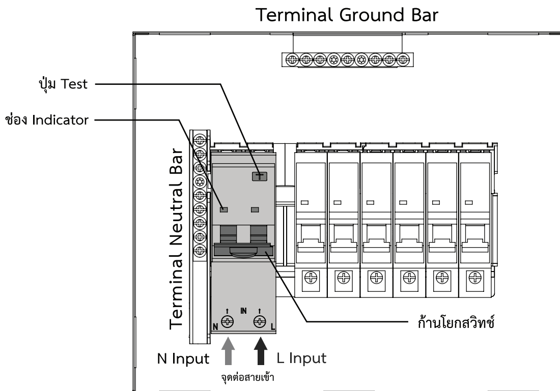
ภาพตัวอย่างการติดตั้งในตู้ Consumer Unit
