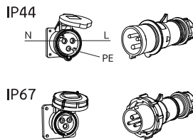
Socket และ Plug 2P+E
