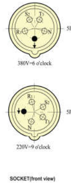
Socket และ Plug 3P+N+E
