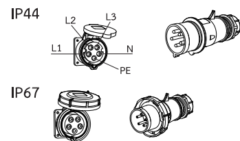
Socket และ Plug 3P+N+E
